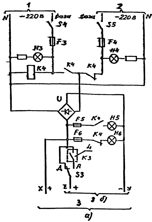
Рис. 12.6. Принципиальная схема питания сети управления постоянным током от выпрямителя. а - при дистанционном, фотоавтоматическом и программном управлении каждым магнитным пускателем, к схемам 12.7, б и 12.7, в; б - при дистанционном управлении каждым пускателем и фотоавтоматическом или программном управлении группой пускателей, к схеме рис. 12.1, б; 1 - основное питание 220 В; 2 - резервное питание 220 В; 3 - постоянный ток 60 В; 4 - замкнут при включении освещения фотоавтоматом.
