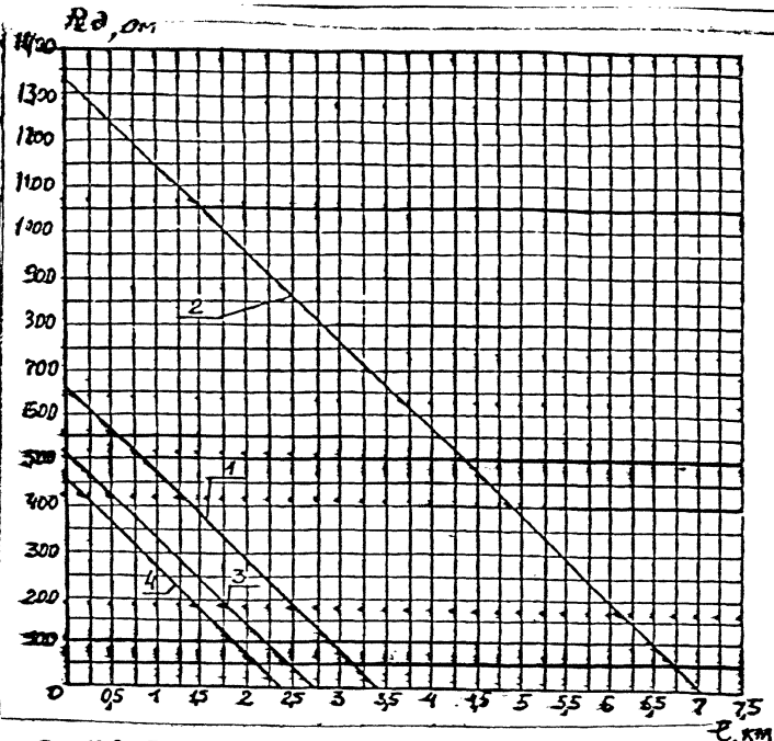
Рис. 2.29. График для определения величины добавочного сопротивления в цепи коммутаторных ламп.
