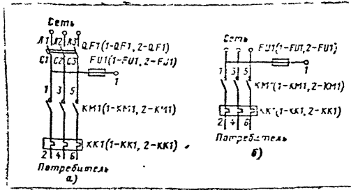
Рис. 16.1. Принципиальные схемы силовых цепей ящиков управления: а - ЯБIII, Я-5III5, ЯБI4I; б - ЯБI3I, ЯБI35. QF1 (1-QF1, 2-QF1) автомат; FU1 (1-FU1, 2-FU1) - предохранитель; КМI (1-КМI, 2-КМI) - пускатель; ККI (1-ККI, 2-ККI) - тепло- вое реле.
