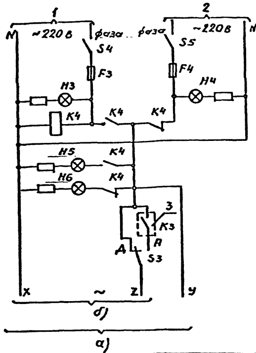
Рис. 12.7. Принципиальная схема питания сети управления переменным током.
