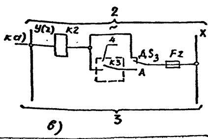
Рис.12.3. Принципиальная схема дистанционного, фотоавтоматического и программного управления освещением по контрольным кабелям с промежуточными реле.
