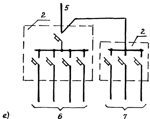
Рис.10.1. Схемы питания НО при отсутствии пиланционного и телемеханического управления. а - непосредственно от ТП; б - от пункта питания НО; в, д - от распределительного пункта без вводного автомата; г, е - от распределительного пункта с вводным автоматом.
