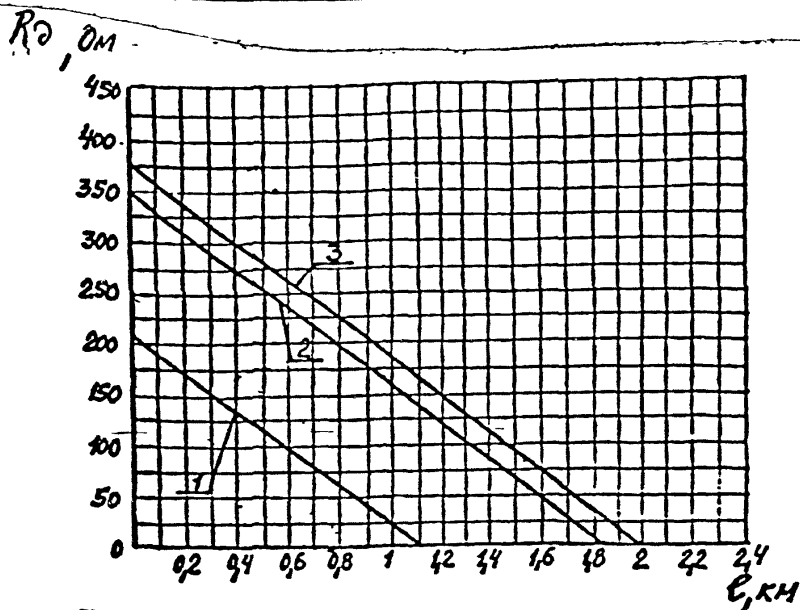
Рис. 12.8. График для определения величины добавочного сопротивления в цепи катушки реле РПУ-2 постоянном токе (при сопротивлении катушек, Ом:
