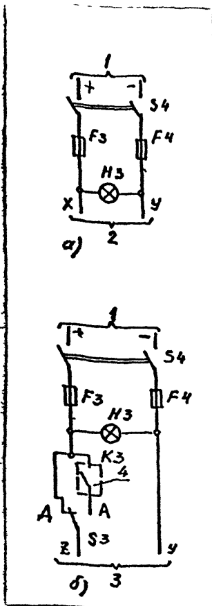
Рис.12.5. Принципиальная схема питания сети управления постоянным током от аккумуляторной батареи.
