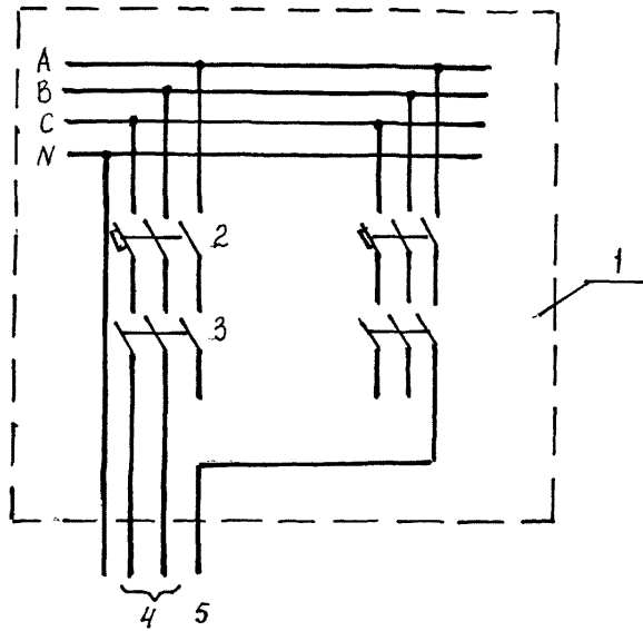
Рис.10.5. Схема включения магнитных пускателей в линию питающей или распределительной сети для раздельного управления вечерними и ночными фазами.
