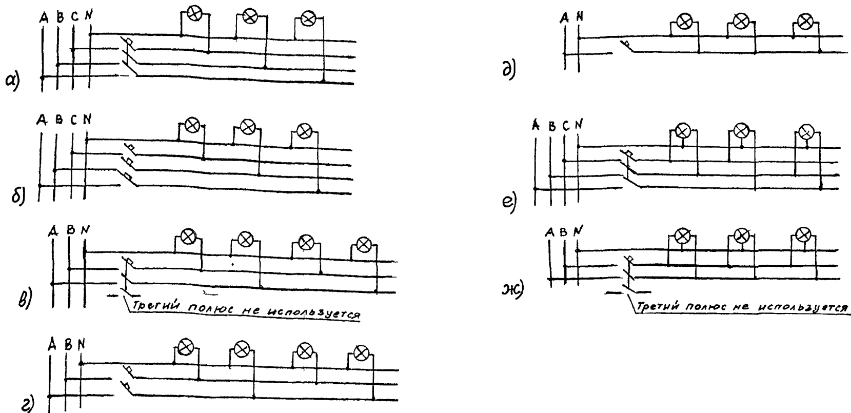
Рис.10.4. Схемы линий распределительной сети. а,б,в,г,д - при питании ОП фазным напряжением 220 В; е,ж - при питании ОП линейным напряжением 380 В. а,б - трехфазная четырехпроводная (3 фазы и нулевой рабочий проводник) с одним трехполюсным или тремя однополюсными автоматами; в,г - двухфазная трехпроводная (2 фазы и нулевой рабочий проводник) с одним трехполюсным или двумя двухполюсными автоматами; д - однофазная двухпроводная; е - трехфазная четырехпроводная (3 фазы и зануляющий проводник); ж - двухфазная трехпроводная (2 фазы и зануляющий проводник).
