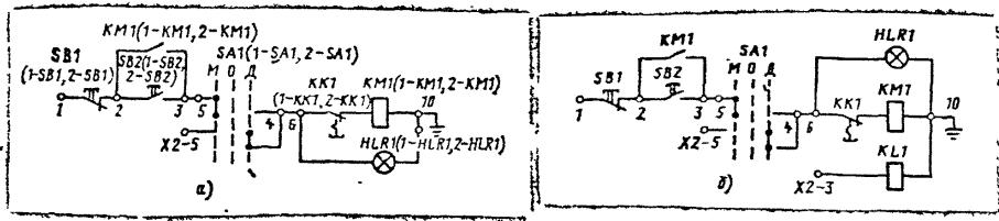
Рис. 16.2. Принципиальные схемы цепей управления ящиков управления: а - ЯБIII, ЯБIII5, ЯБI35; б - ЯБI4I. SA1 (1-SA1, 2-SA1) - предохранитель; HLR1 (1-HLR1, 2-HLR1) - лампа; SB1 (1-SB1, 2-SB1), SB2 (1-SB2, 2-SB2) - кнопки управления; КМI - промежуточное реле.
