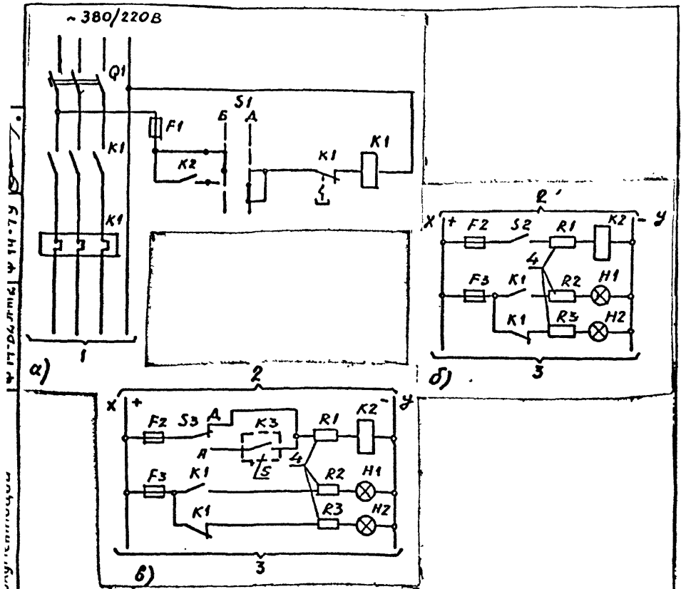
Рис. 12.1. Принципиальная схема дистанционного, фотоавтоматического и программного управления освещением по свободным жилам телефонных кабелей.
