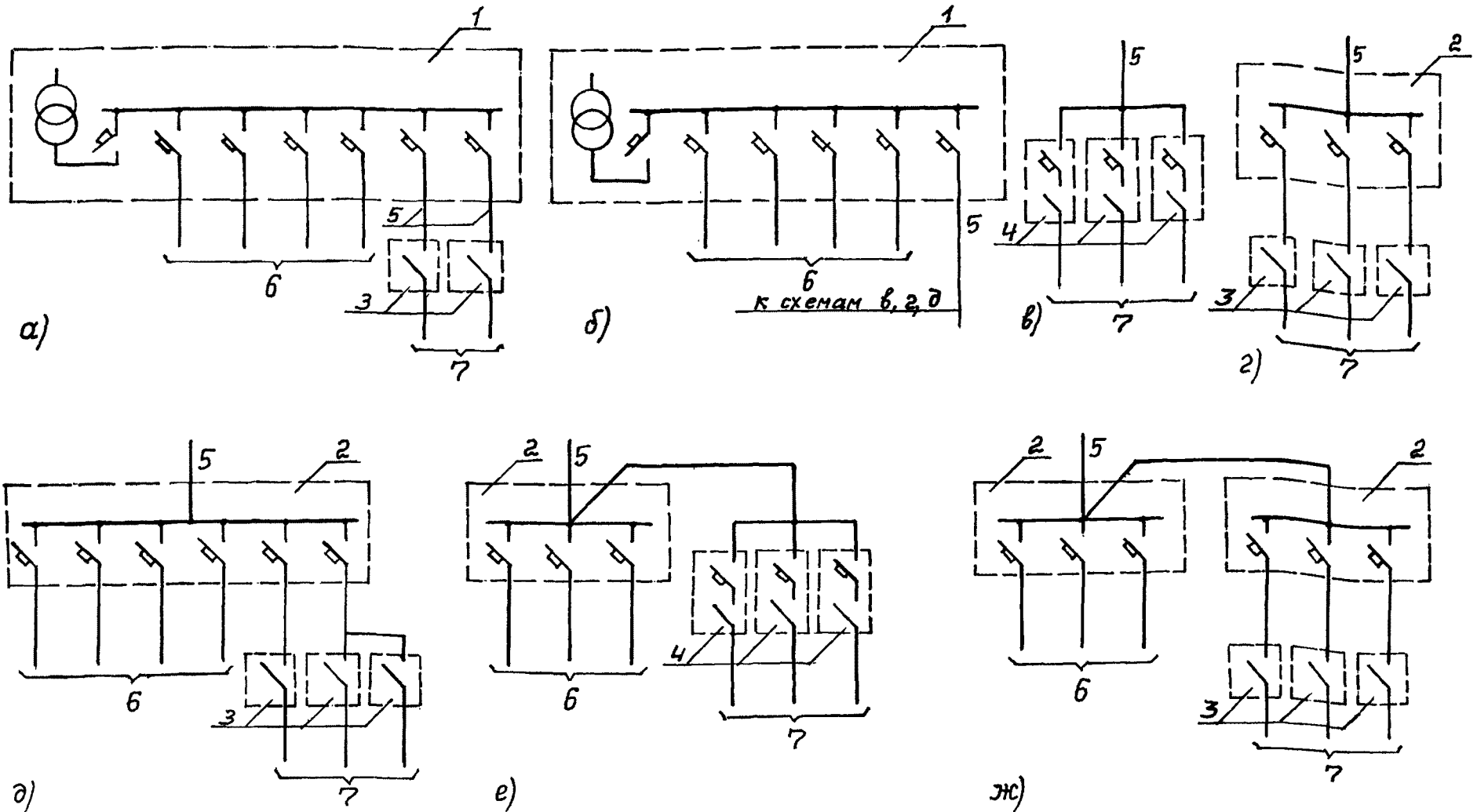
Рис.10.3. Схемы питания НО при дистанционном или телемеханическом управлении с магнитными пускателями в линиях распределительной сети. а - непосредственно от ТП; б - от пунктов питания НО; в - от ящиков с автоматом и магнитным пускателем (или от шита управления); г - от распределительного пункта и ящиков управления с магнитным пускателем; д - от распределительного пункта, общего для НО и других потребителей и ящиков управления с магнитным пускателем; е - общей линией питающей сети с другими потребителями и ящиков управления с автоматом и магнитным пускателем (или от шита управления); ж - общей линией питающей сети с другими потребителями от распределительного пункта и ящиков с магнитным пускателем.
