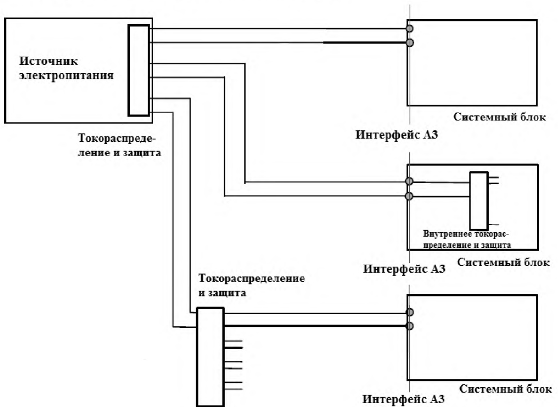
Рисунок А.1 – Примеры расположения интерфейса А3
