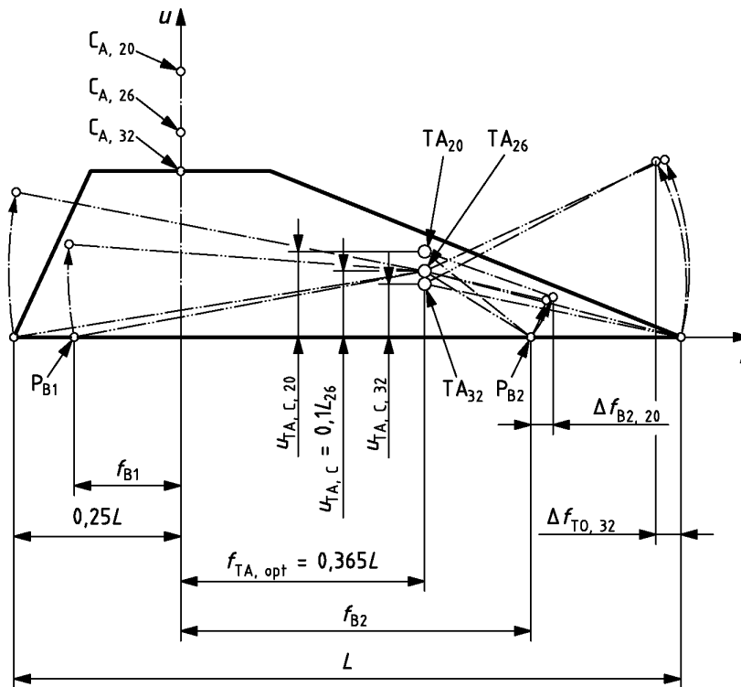
Рисунок 24 – Иллюстрация влияния постоянного компромиссного смещения u_{TA,C} оси наклона TA платформы стопы на A-P смещение \Delta f в узле стопы при разной длине узла стопы L [см. 3.8.2, перечисление с) 2)]
