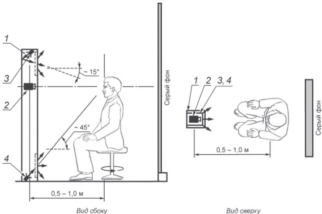
1 — консоль регистрации; 2 — камера; 3 — верхний осветитель; 4 — нижний осветитель
