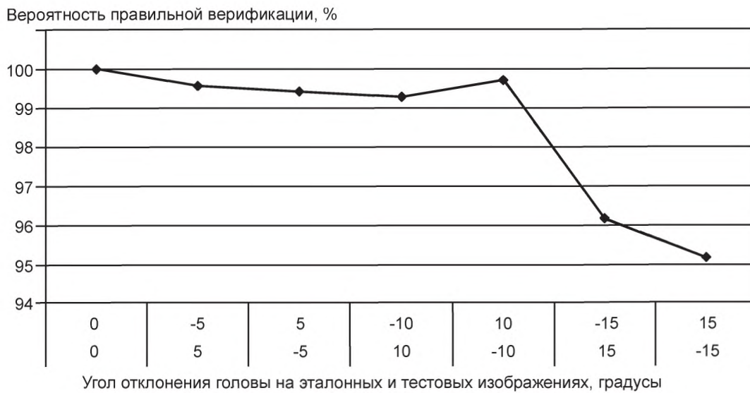
Рисунок D.8 — Зависимость вероятности правильной верификации от угла отклонения головы при вероятности ложного допуска 0,1 %
