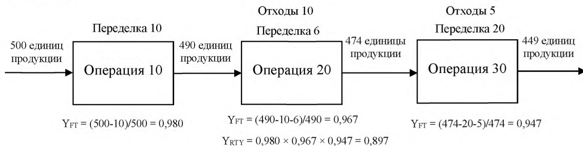
Рисунок 3 – Пример вычисления вероятности штучного сквозного выхода
