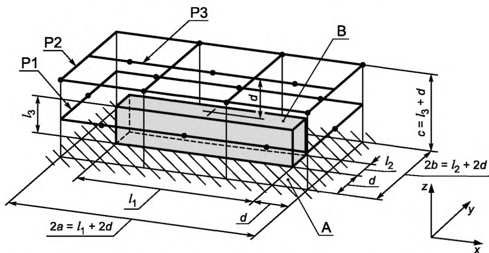
Рисунок С.8 — Пример измерительной поверхности, точек установки микрофонов и траекторий сканирования при испытаниях высоких машин с малой площадью основания ( l_1 \leq d, l_2 \leq d, 2d < l_3 \leq 5d )
