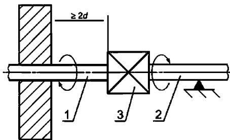
d – наружный диаметр; 1 – труба; 2 – труба; 3 – испытуемый образец
