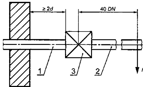
Рисунок 6 – Схема испытания устройства контроля пламени на изгиб
