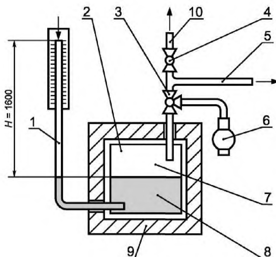
1 – трубка со шкалой в миллиметрах; 2 – термически изолированный сосуд под давлением; 3 – трехходовой кран; 4 – кран; 5 – патрубок для присоединения образца для испытаний; 6 – компрессор; 7 – воздушный объем 1 дм 3 ; 8 – вода; 9 – теплоизоляция; 10 – напорная трубка
