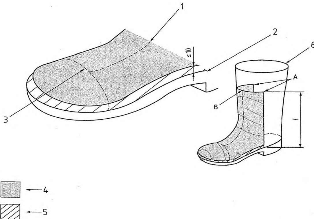
1 – геометрическая ось обуви; 2 – линия кромки; 3 – спинка подноски; 4 – защитная область; 5 – дополнительная защитная область для обуви уровней защиты 3 и 4; 6 – верхний край верха обуви
