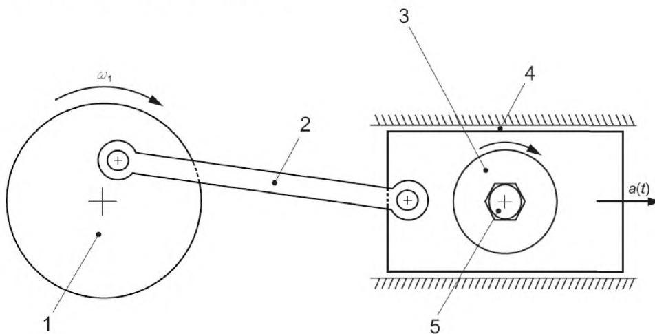
1 – вращающийся диск; 2 – шатун; 3 – поворотный стол, управляемый шаговым двигателем; 4 – скользящая или воздушная опора; 5 – калибруемый преобразователь; a(t) – ускорение; \omega_1 – угловая частота
