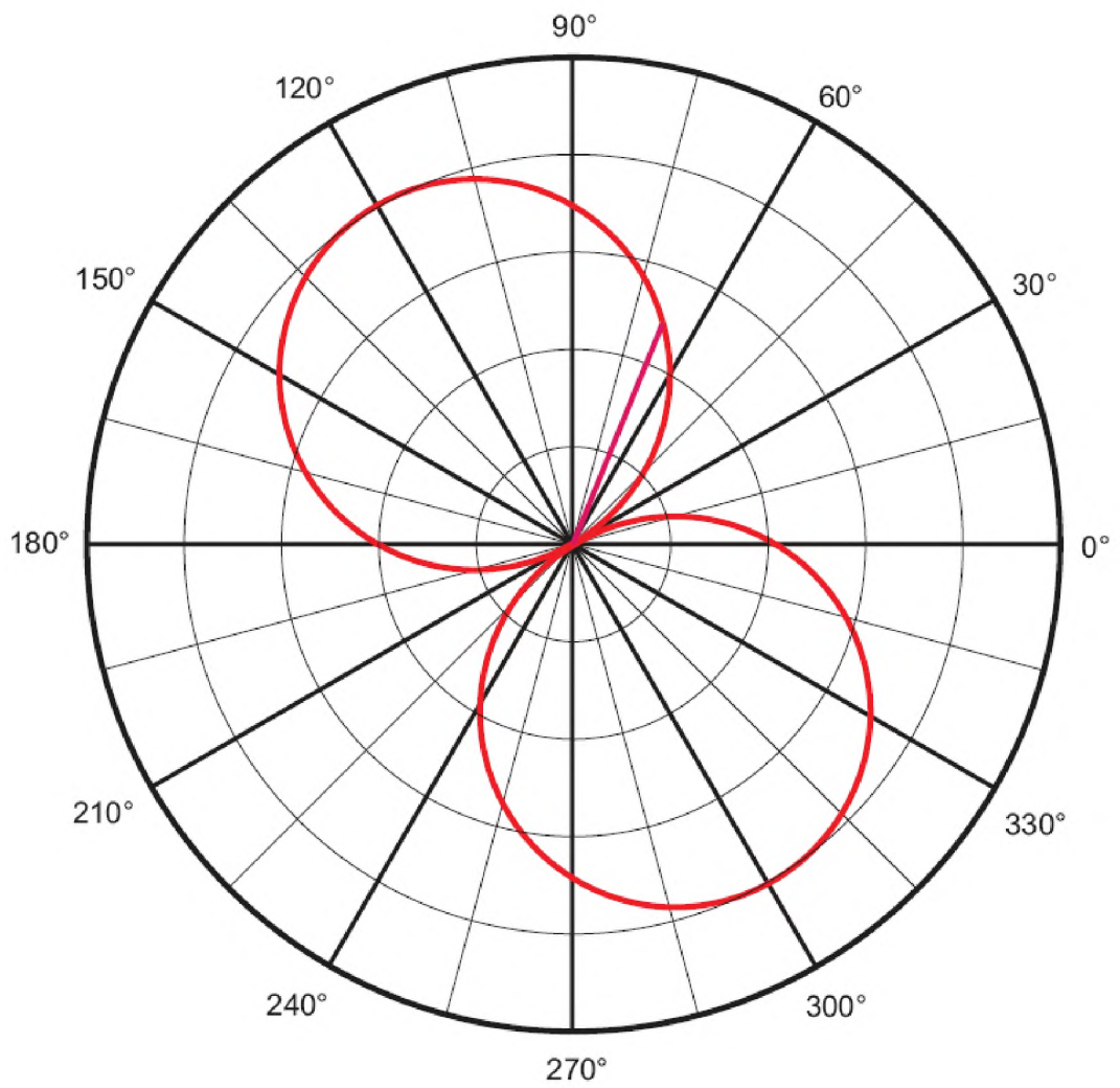
Рисунок А.2 – Типичная теоретическая кривая коэффициента поперечного преобразования в полярной системе координат как функция угла в плоскости, перпендикулярной к оси чувствительности преобразователя
