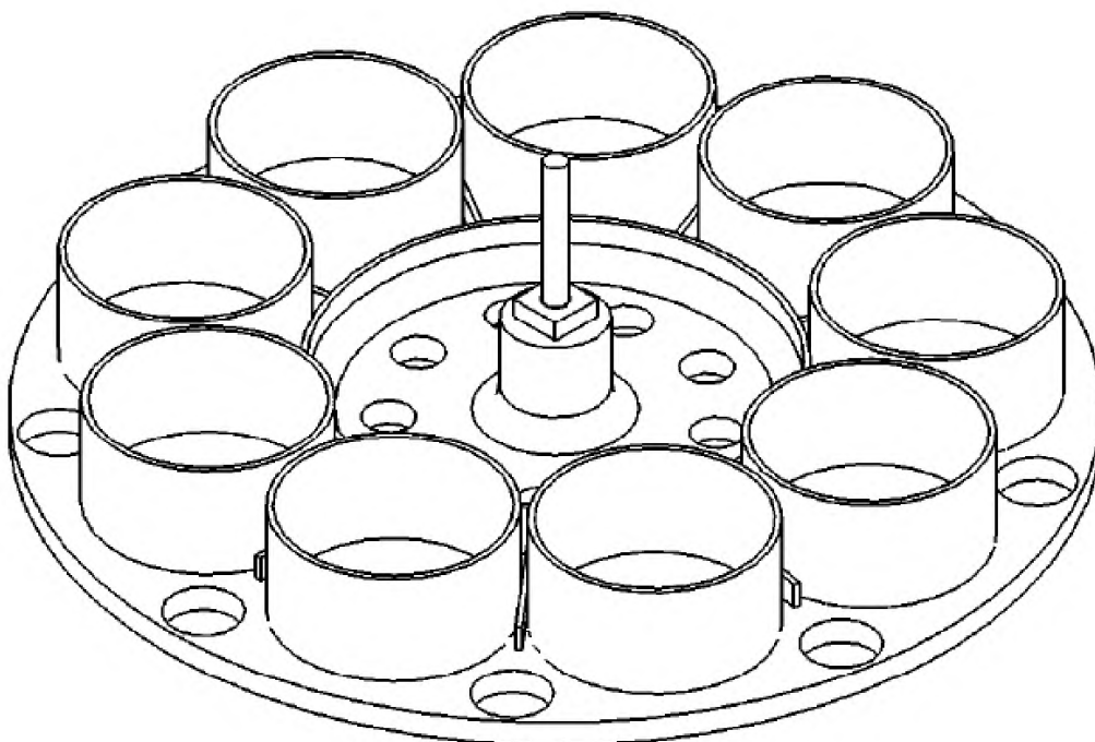
b – Трехмерное изображение алюминиевой полки Рисунок 1, лист 2
