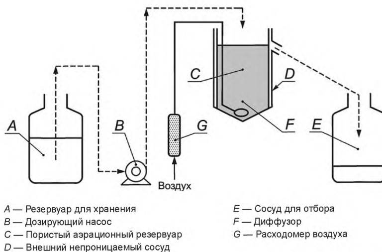
Рисунок 2 — Оборудование, применяемое для оценки биоразложения
