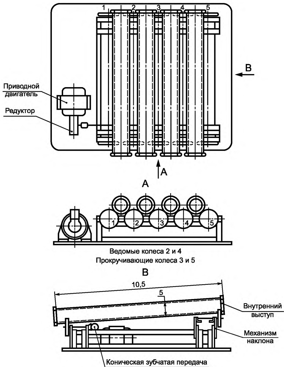
Рисунок 3 — Вращающиеся трубы
