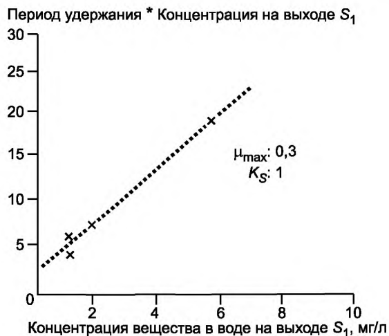
Рисунок Д.2 — Линия регрессии, период удержания S_1 от S_1 , T = 5 \text{ } ^\circ\text{C}
