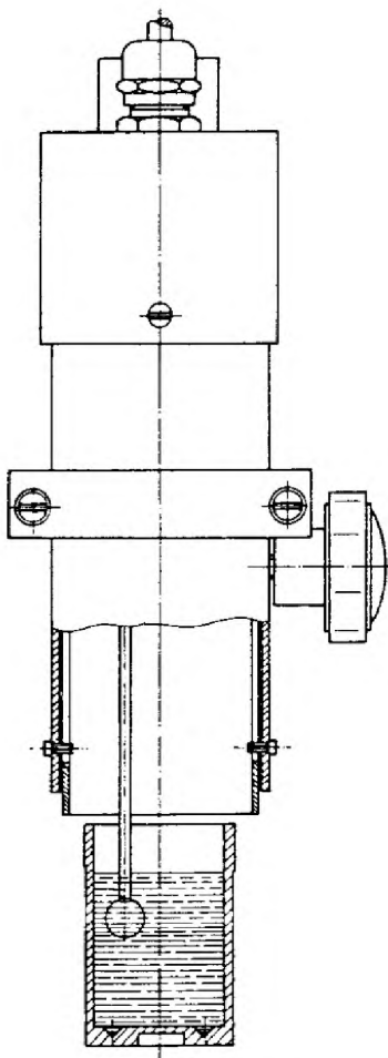
Рисунок А.2 – Сосуд для испытуемой пробы
