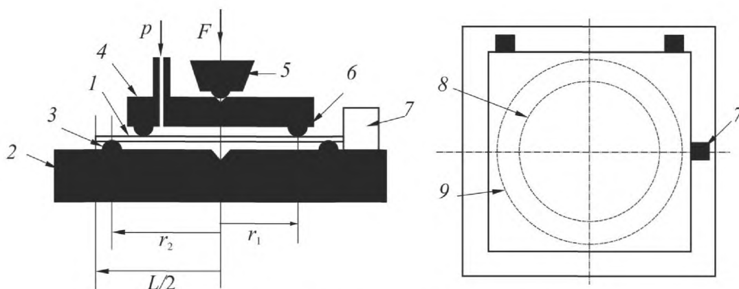
Рисунок 2 – Нагрузочное устройство
