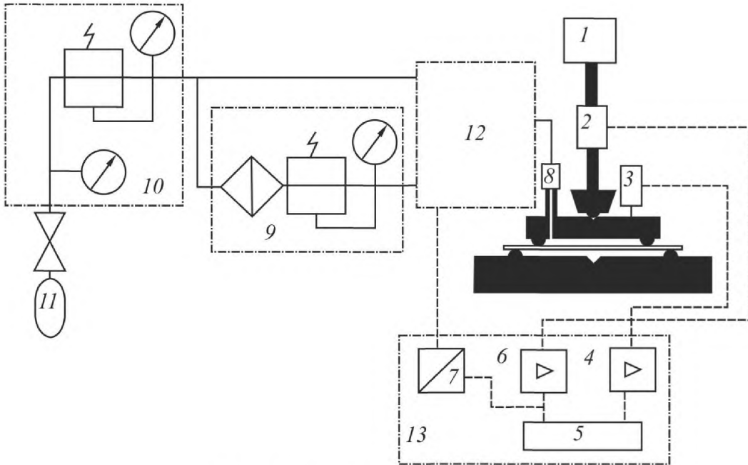
Рисунок А.2 – Схема системы контроля
