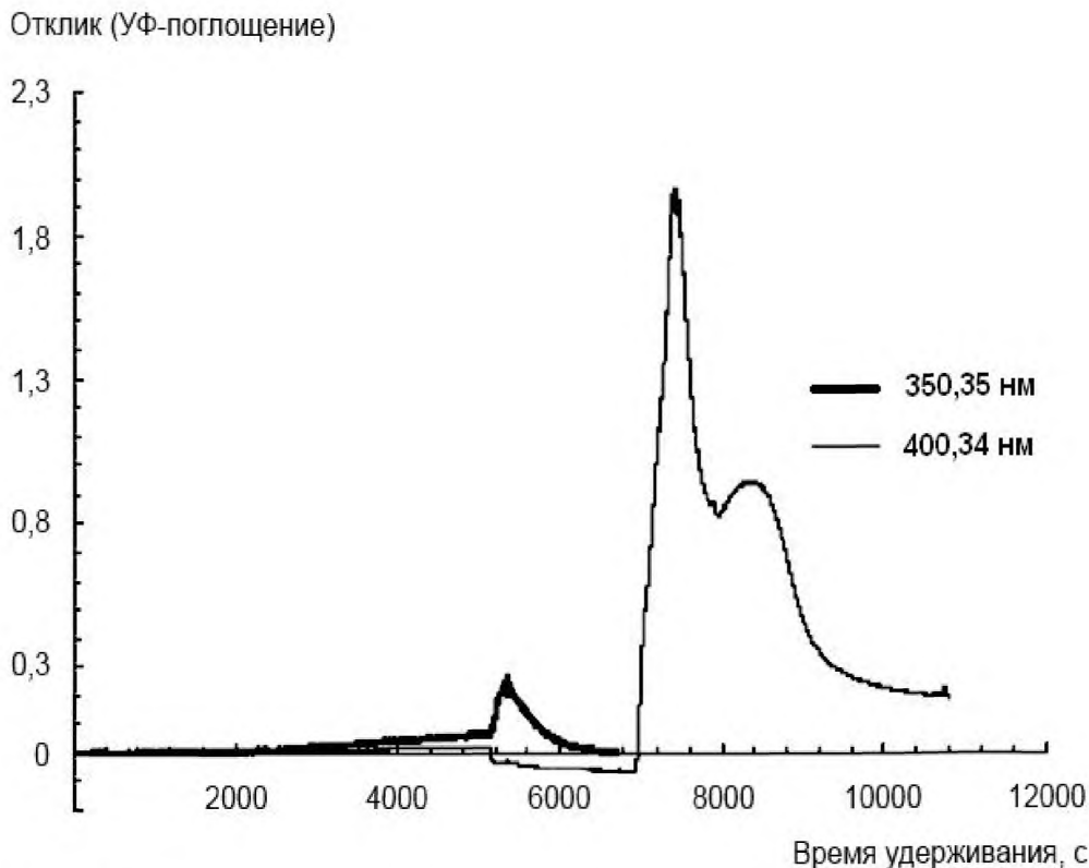
Рисунок 3 – Хроматограмма, показывающая пики удерживания фракций нафтеновых ароматических и полярных ароматических соединений
