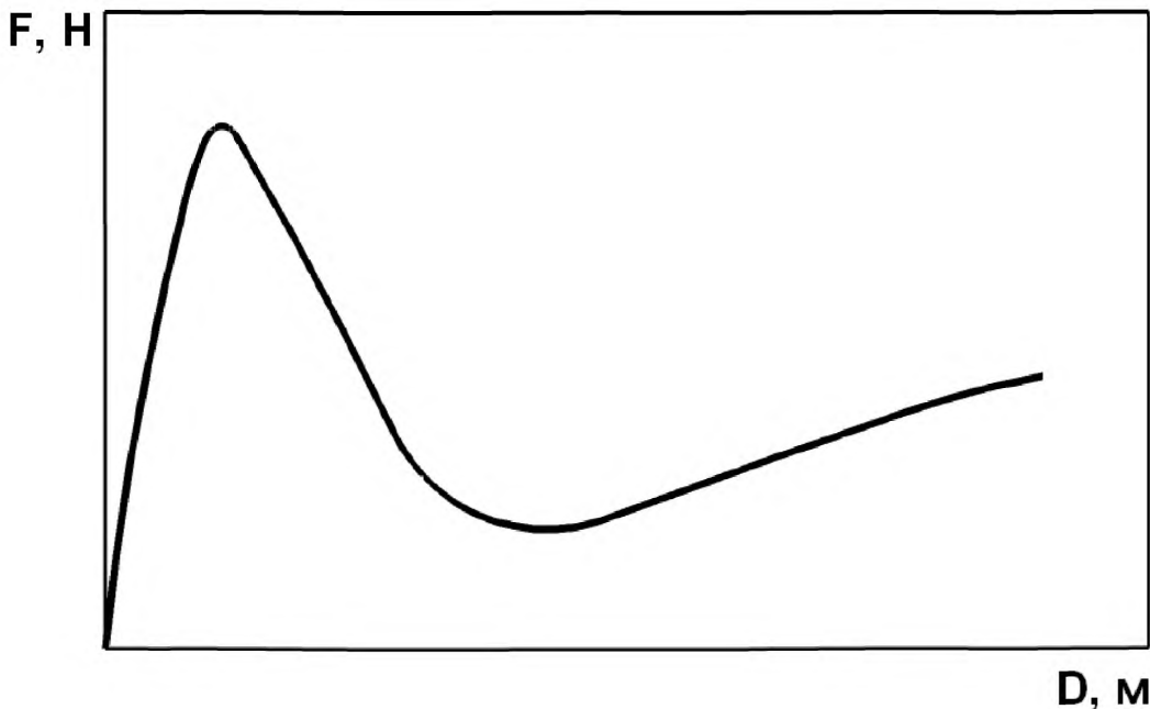
Рисунок А.1 – Зависимость силы от удлинения
