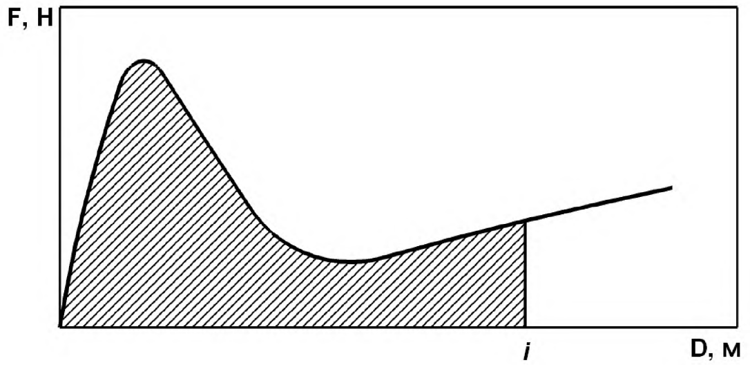
Рисунок А.2 – Энергия при заданном удлинении
