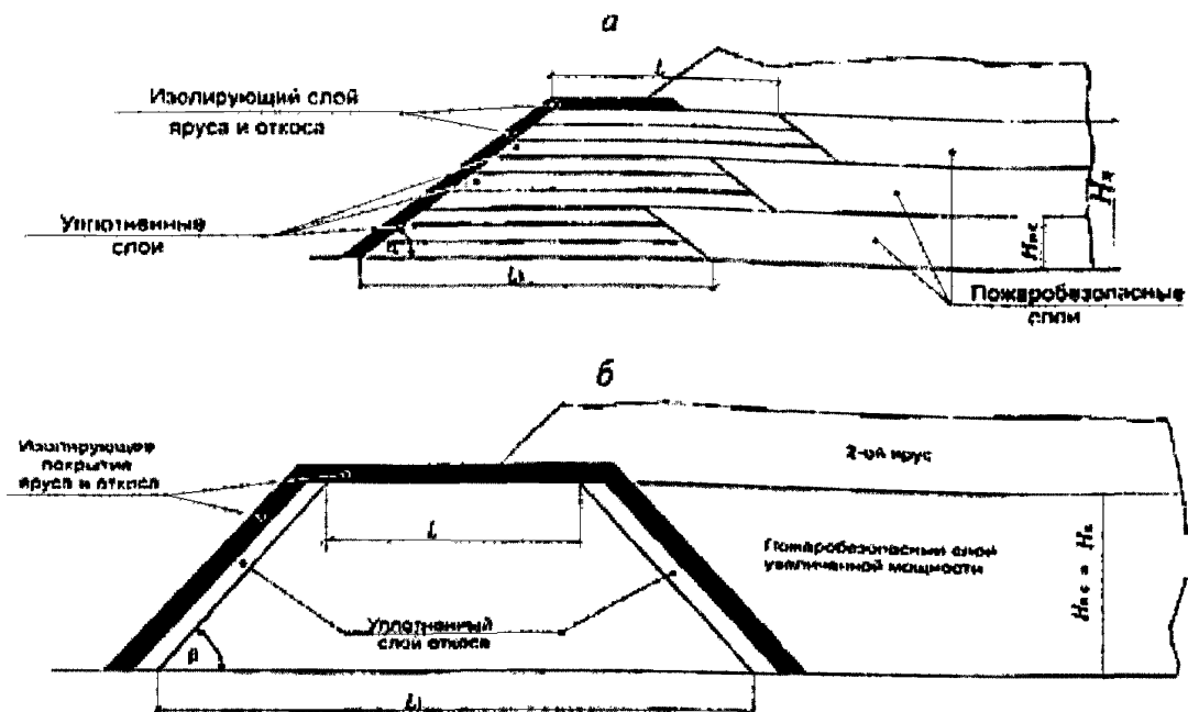
Рис. 2. Периферийный способ формирования породных отвалов: a — формирование отвала пожаробезопасными слоями; б — формирование отвала пожаробезопасными слоями увеличенной мощности
