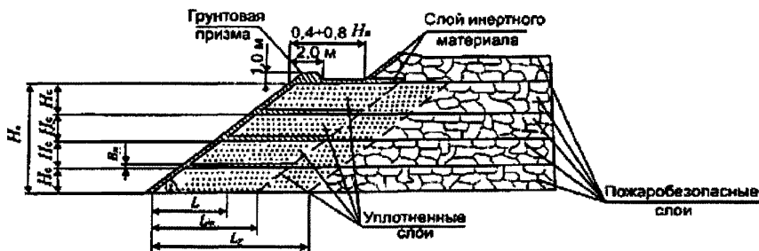
Рис. 1. Схема формирования яруса
