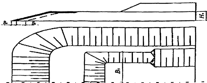
Рис. 2. Формирование отвала пожаробезопасными слоями увеличенной мощности
