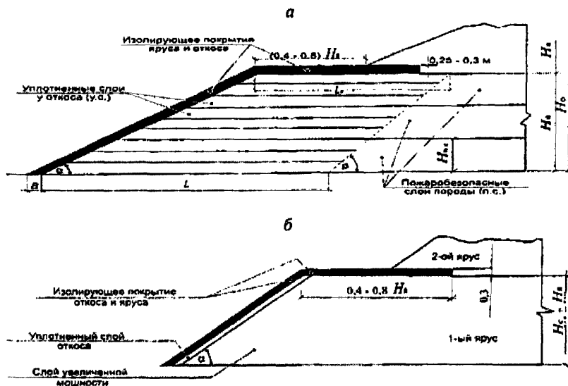
Рис. 1. Фронтальный способ формирования породных отвалов: а — формирование отвала пожаробезопасными слоями; б — формирование отвала пожаробезопасными слоями увеличенной мощности
