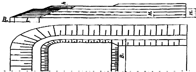
Рис. 1. Формирование отвала пожаробезопасными слоями
