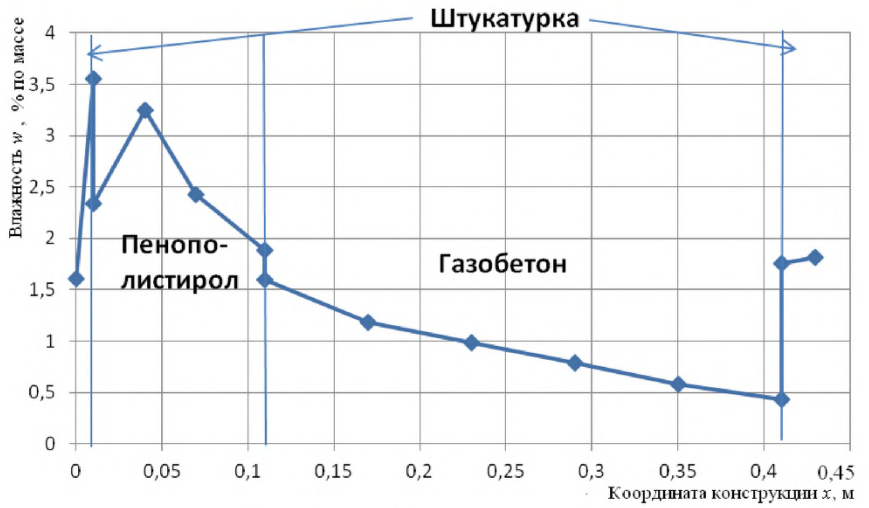
Рисунок Г.1 – Распределение влажности внутри конструкции
