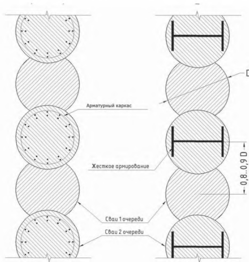
Рисунок 1 – Буросекущие сваи, схема армирования
