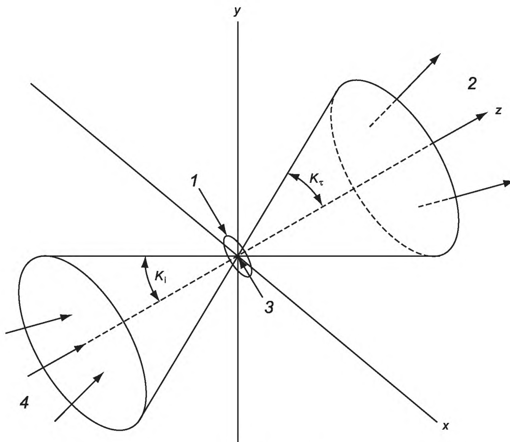
1 — измерительная апертура; 2 — исходящий поток излучения; 3 — точка 0; 4 — падающий поток излучения; K_i — половина угла конуса диффузного падающего потока излучения; K_r — половина угла конуса диффузного исходящего потока излучения
