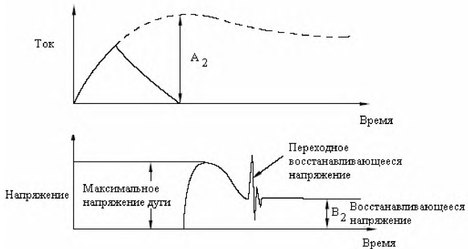
Рисунок С.2 – Отключение высоковольтного предохранителя при появлении дуги после достижения максимального значения тока
