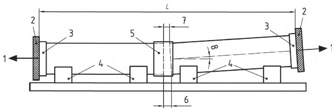
1 – осевое давление, воздействующее на образец; 2 – оснастка испытательного стенда; 3 – торцевая заглушка; 4 – опоры; 5 – испытуемое соединение; 6 – общий вырыв; 7 – вырыв; 8 – угловое смещение; L – общая эффективная длина
