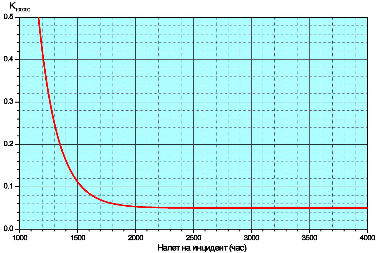
Рисунок 2 — Зависимость K_{100000} от налета на инцидент для самолетов ГА РФ
