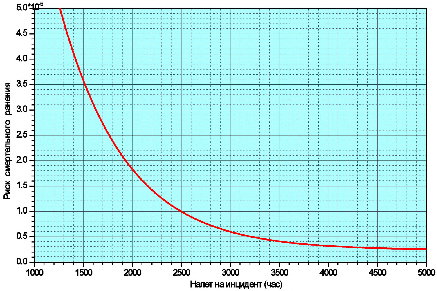
Рисунок 3 — Зависимость РСР от налета на инцидент для вертолетов ГА РФ
