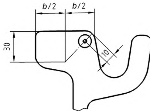
Рисунок 3 — Расположение образца для определения механических свойств
