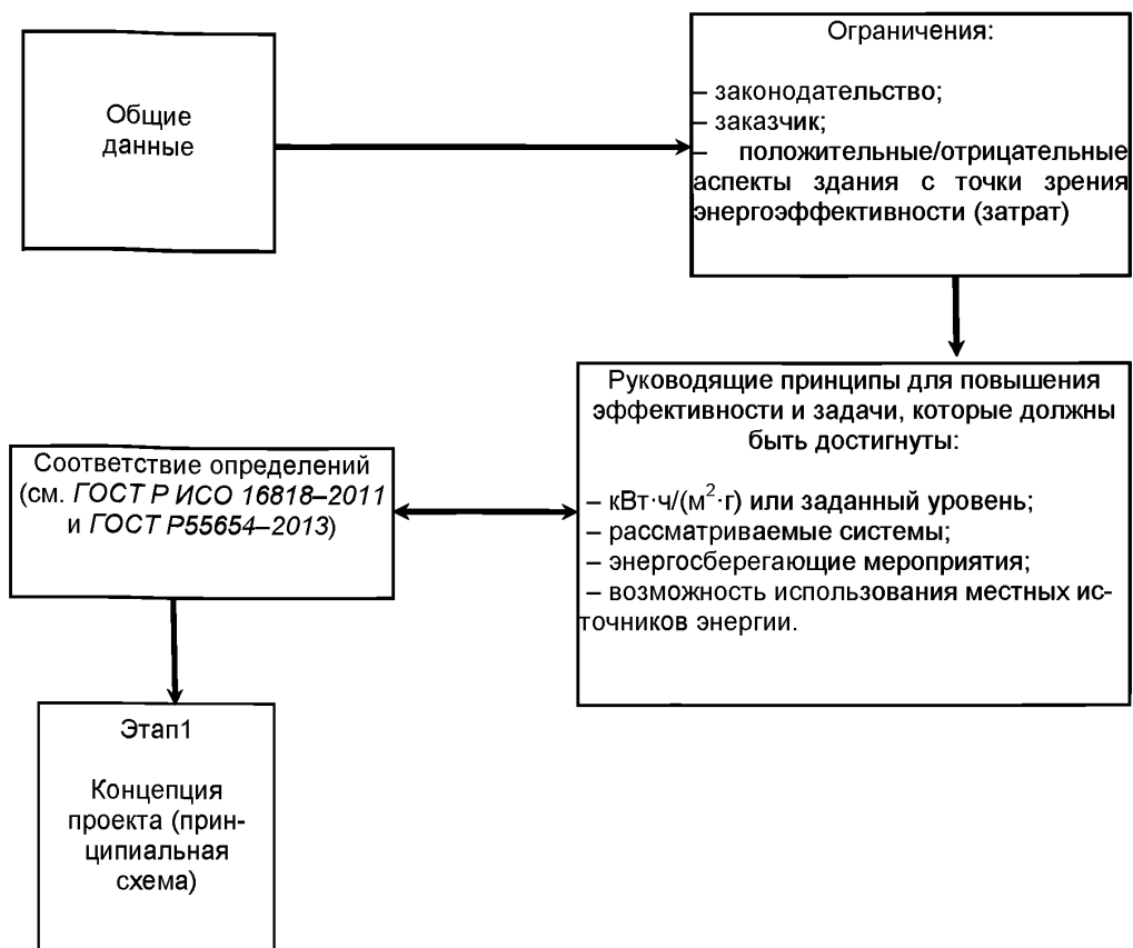
Рисунок А.1 – Блок-схема процесса проектирования энергоэффективности здания
