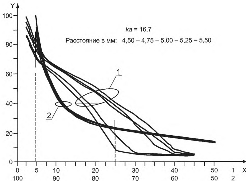
Рисунок D.1 — Линии равных давлений типовой физиотерапевтической лечебной головки малой геометрической площади ( ka = 17 )
