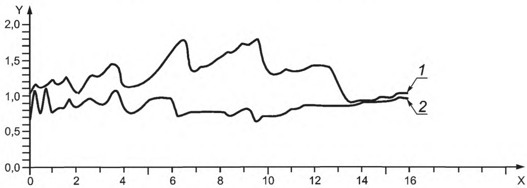
X: z/\lambda Y: A_{BCS} (мм 2 ) (1 — по стандарту FDA; 2 — по стандарту МЭК)
