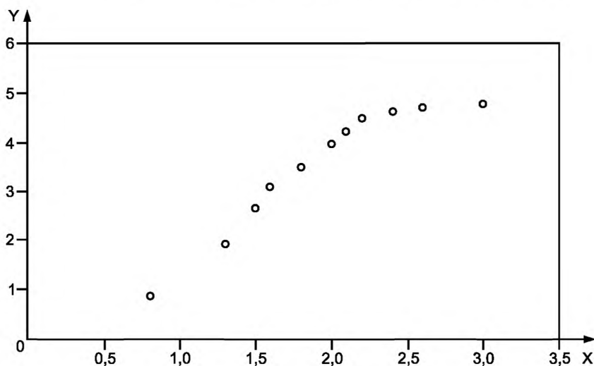
Рисунок I.2 — Измеренная мощность, прошедшая через апертуры различного диаметра, для лечебной головки с частотой 1 МГц
