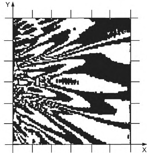
Рисунок D.1 — Линии равных давлений типовой физиотерапевтической лечебной головки малой геометрической площади ( ka = 17 )
