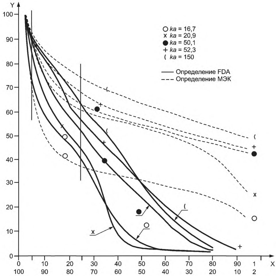
X: Процент ограничения (1 — по стандарту FDA; 2 — по стандарту МЭК); Y: Соответствующее значение A_{BCS} (мм 2 )
