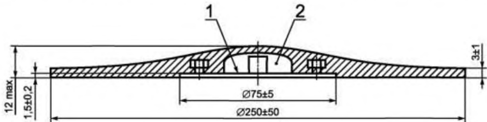
1 – тонкая металлическая пластина для установки акселерометра; 2 – полость для установки акселерометра
