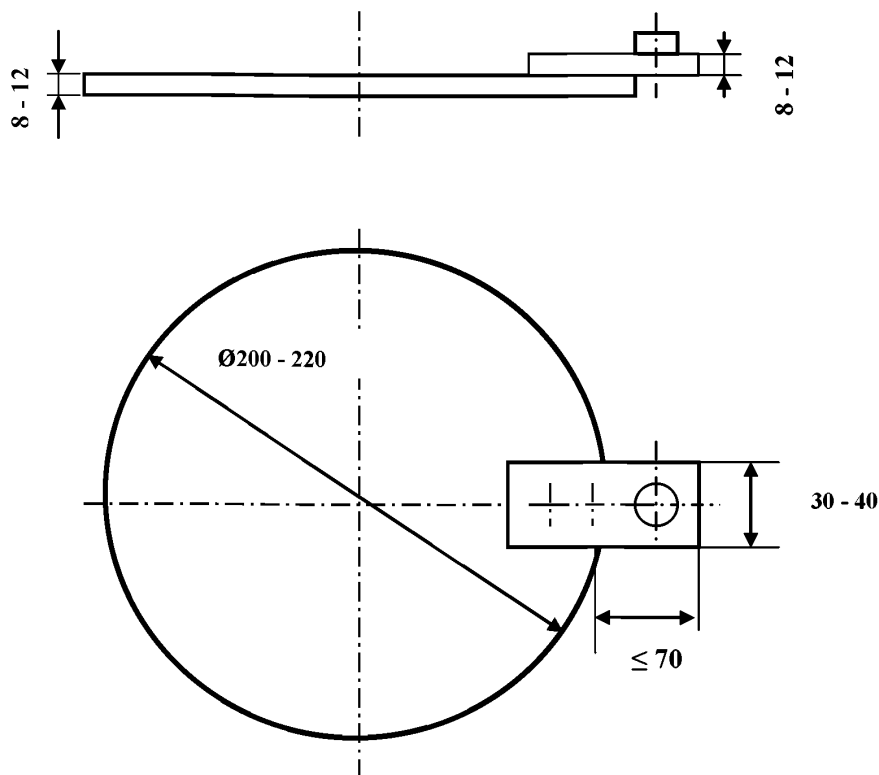
Рисунок 4 - Жесткий установочный диск
