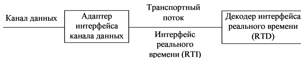
Р и с у н о к 1 – Схема интерфейса реального времени (RTI)
