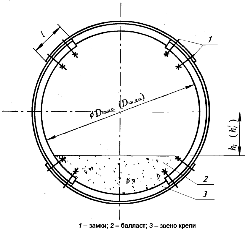
1 – замки; 2 – балласт; 3 – звено крепи
