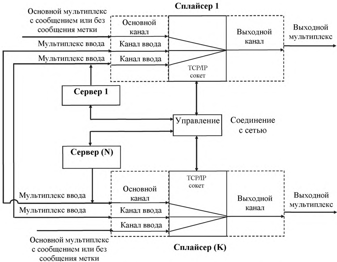
Р и с у н о к 1 – Конфигурация с несколькими серверами и сплайсерами
