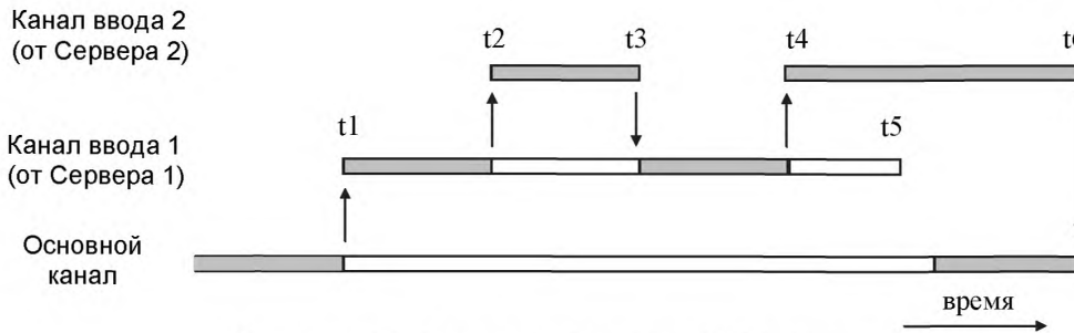
Рисунок 2 – Операция флага OverridePlaying
