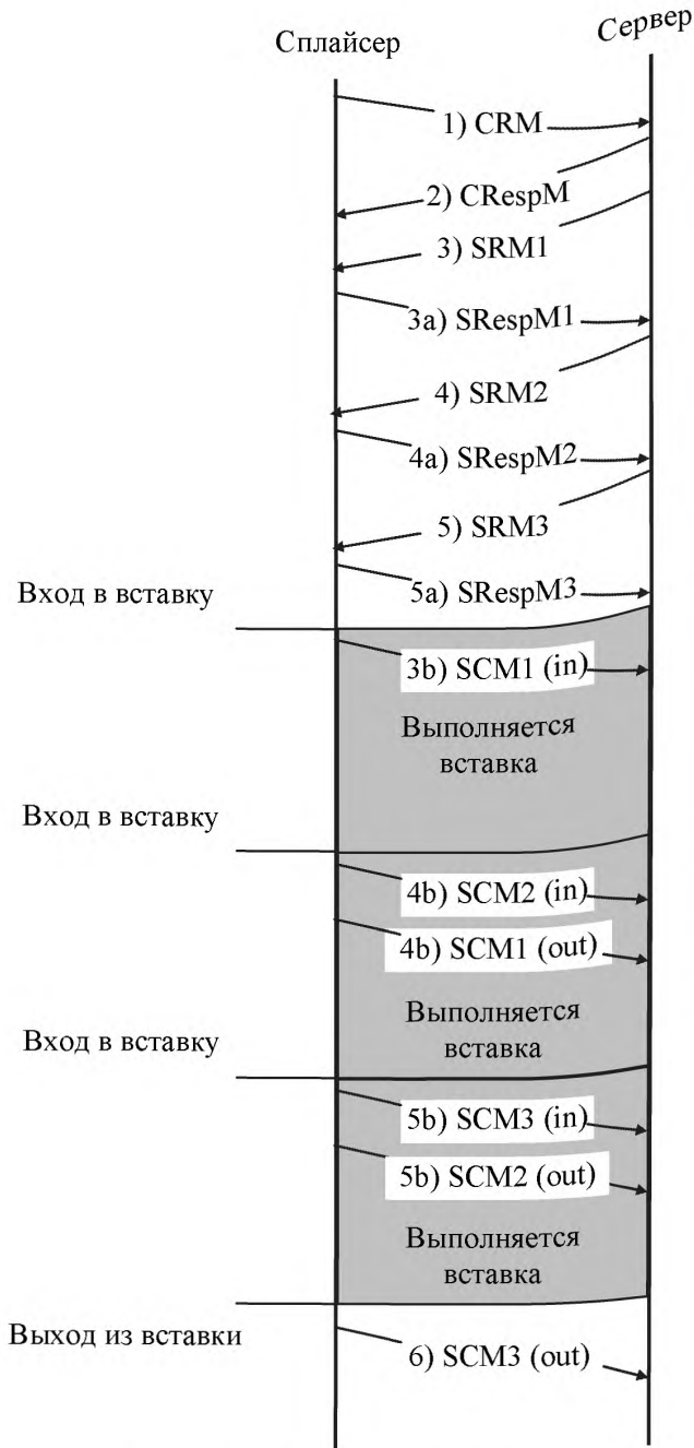
Рисунок 4 – Сценарий вставки нескольких событий
