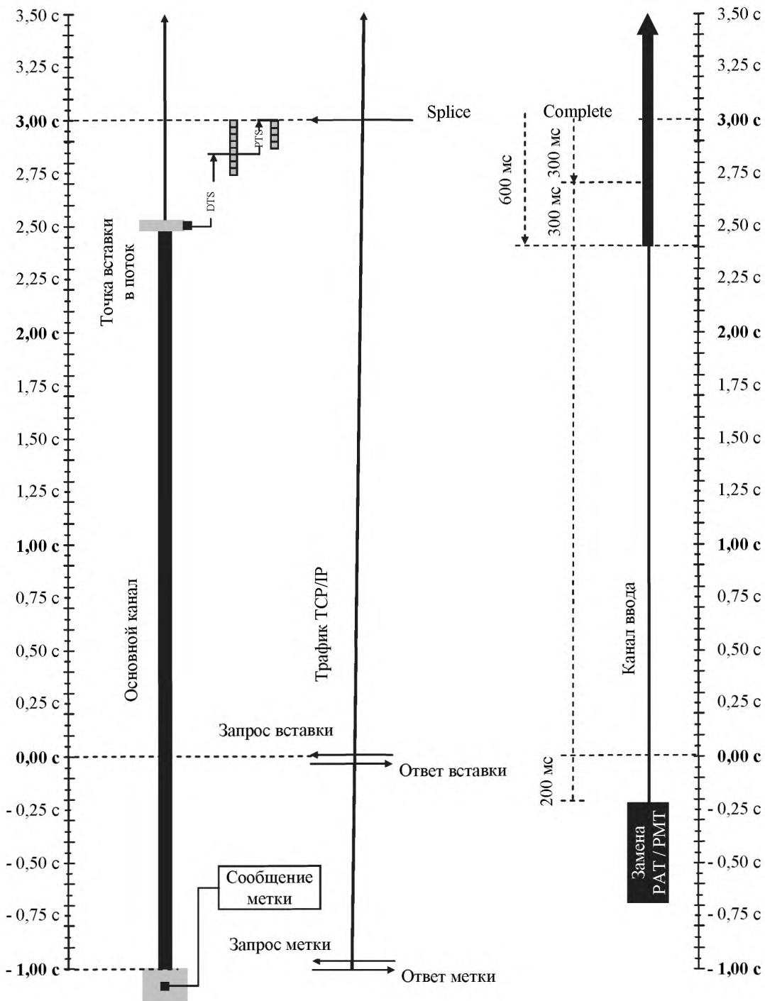
Рисунок 5 – Временная шкала иницирования вставки рекламы
