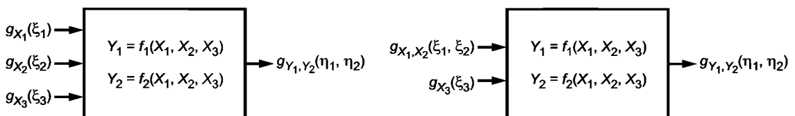
Рисунок 1 — Трансформирование распределений для модели с N = 3 входными величинами и m = 2 выходными величинами, когда входные величины X_1, X_2 и X_3 взаимно независимы (слева) и когда X_1 и X_2 взаимно зависимы (справа)
