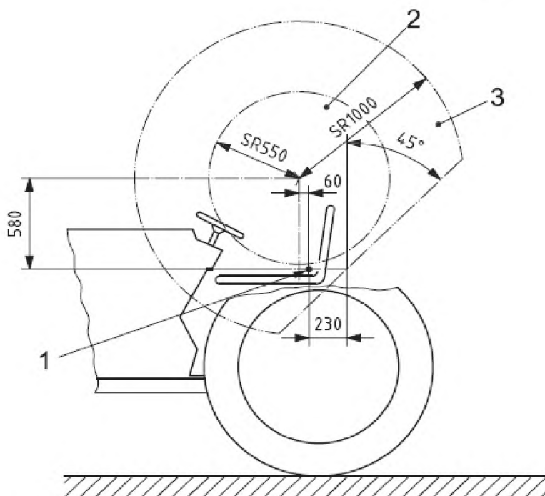
Рисунок 1 – Зона досягаемости рук оператора
