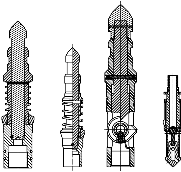
Рисунок Е.5 — Защелки
