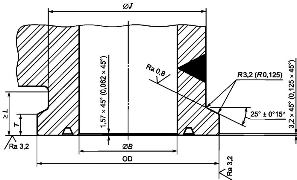
Рисунок 3 — Цельные бугельные соединения типа 16В и 16ВХ
