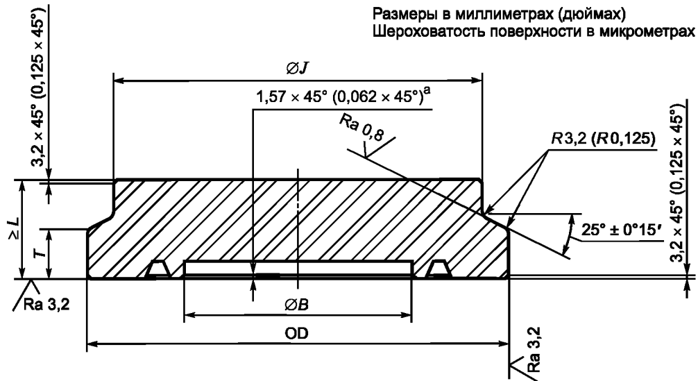
Рисунок 3 — Цельные бугельные соединения типа 16В и 16ВХ
