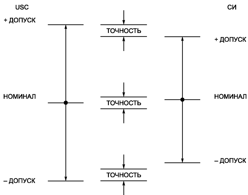
а) Двухсторонний допуск
