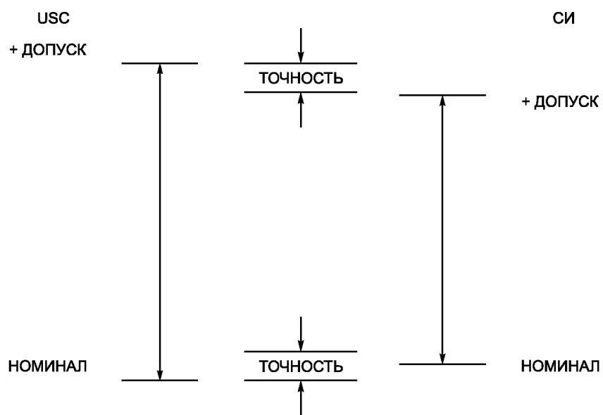
б) Односторонний допуск
