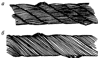
Рис. 2. Сочетание обрывов проволок с их износом: а — в канате крестовой свивки; б — в канате односторонней свивки
