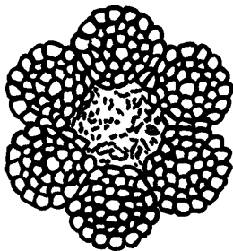
Рис. 8. Уменьшение площади поперечного сечения проволоки (интенсивная внутренняя коррозия)
