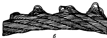
Рис. 12. Выдавливание проволок прядей: а — в одной пряди; б — в нескольких прядях
