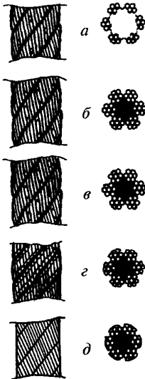
Рис. 5. Износ наружных проволок каната крестовой свивки: а — небольшие лыски на проволоках; б — увеличенная длина лысок на отдельных проволоках; в — удлинение лысок в отдельных проволоках при заметном уменьшении диаметра проволок; г — лыски на всех проволоках, уменьшение диаметра каната; д — интенсивный износ всех наружных проволок каната (уменьшение диаметра проволок на 40 %)
