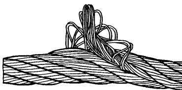
Рис. 11. Выдавливание сердечника
