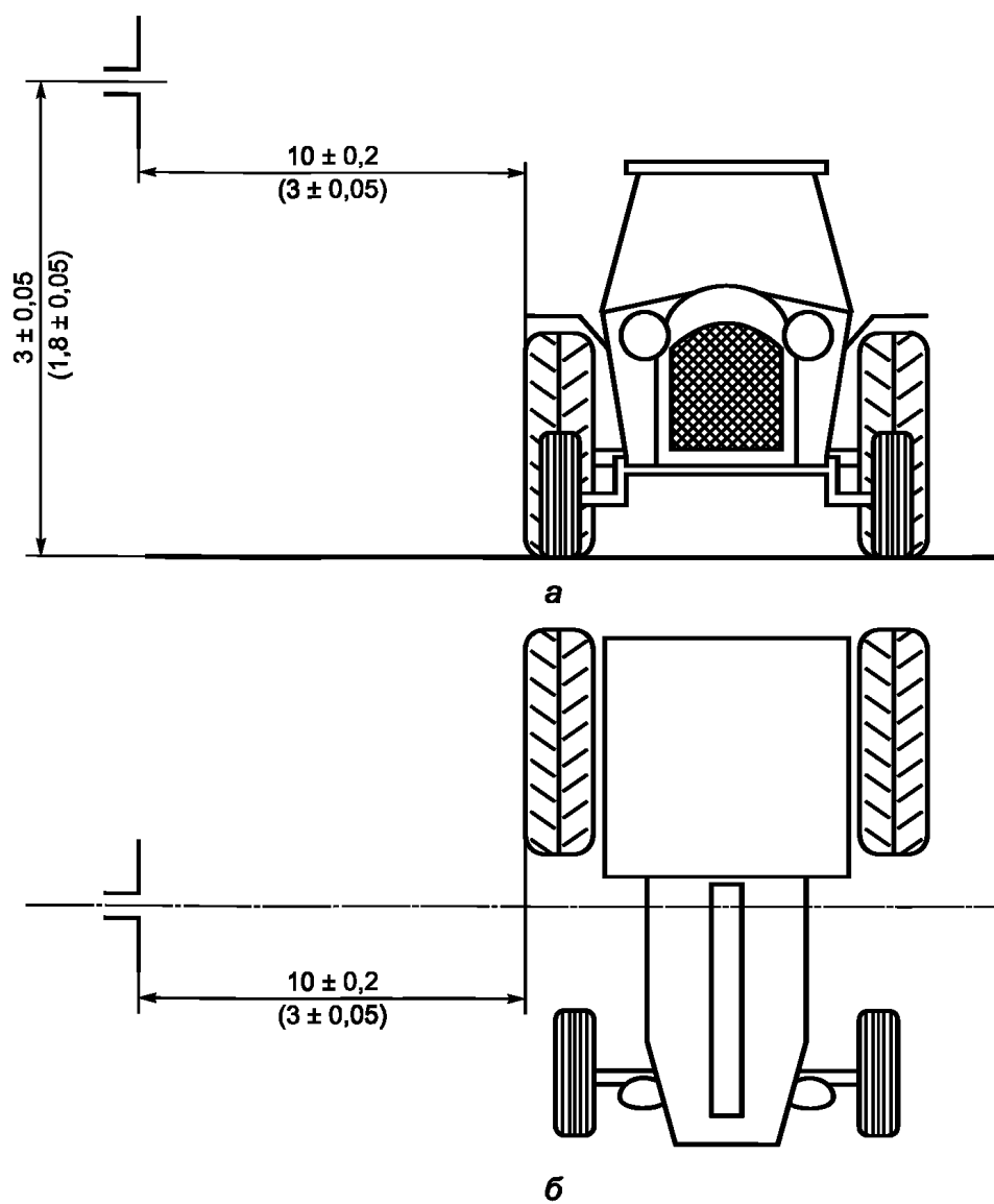
a — положение симметричной вибраторной антенны для измерения вертикальной компоненты излучения; b — положение симметричной вибраторной антенны для измерения горизонтальной компоненты излучения
