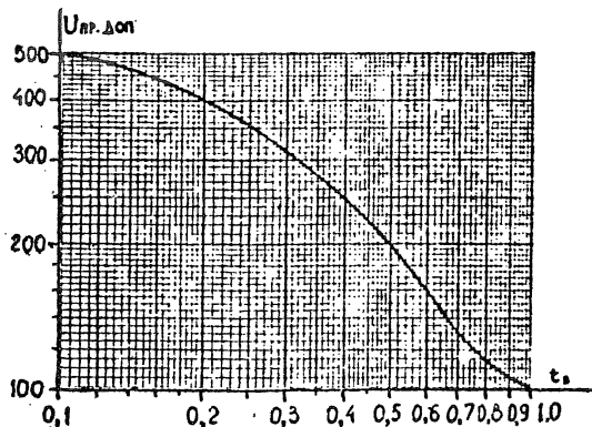
Рис. III.I. Зависимость U_{пр. доп} от t_s .
