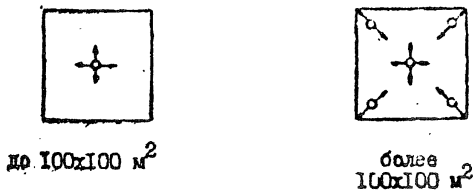
Рис.4.1. Расположение центров зондирования и направления полуразросов установок ВЭЗ
