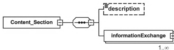
Рисунок 12 — Графическое представление элемента ADM-матрицы Content_Section
