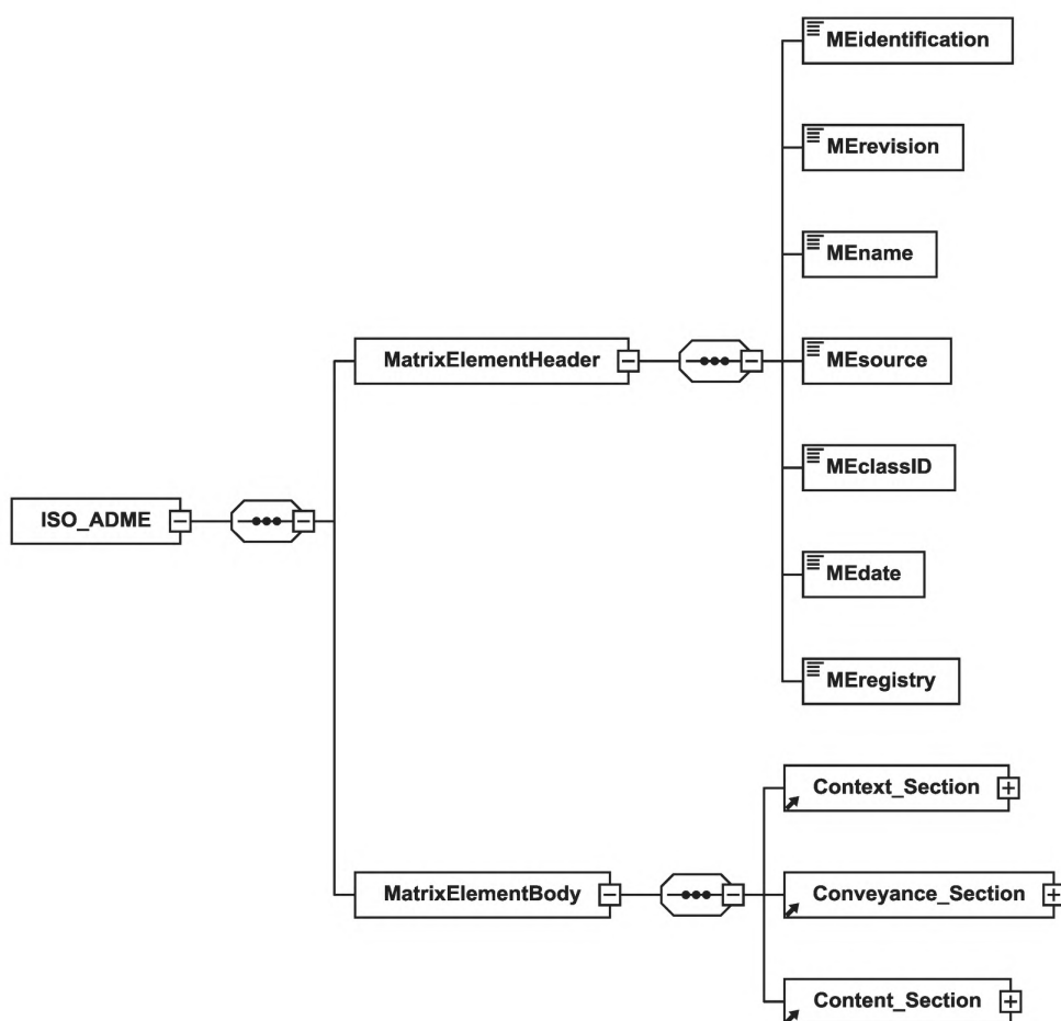
Рисунок 9 — Графическое представление элемента ADM-матрицы MatrixElementHeader и MatrixElementBody
