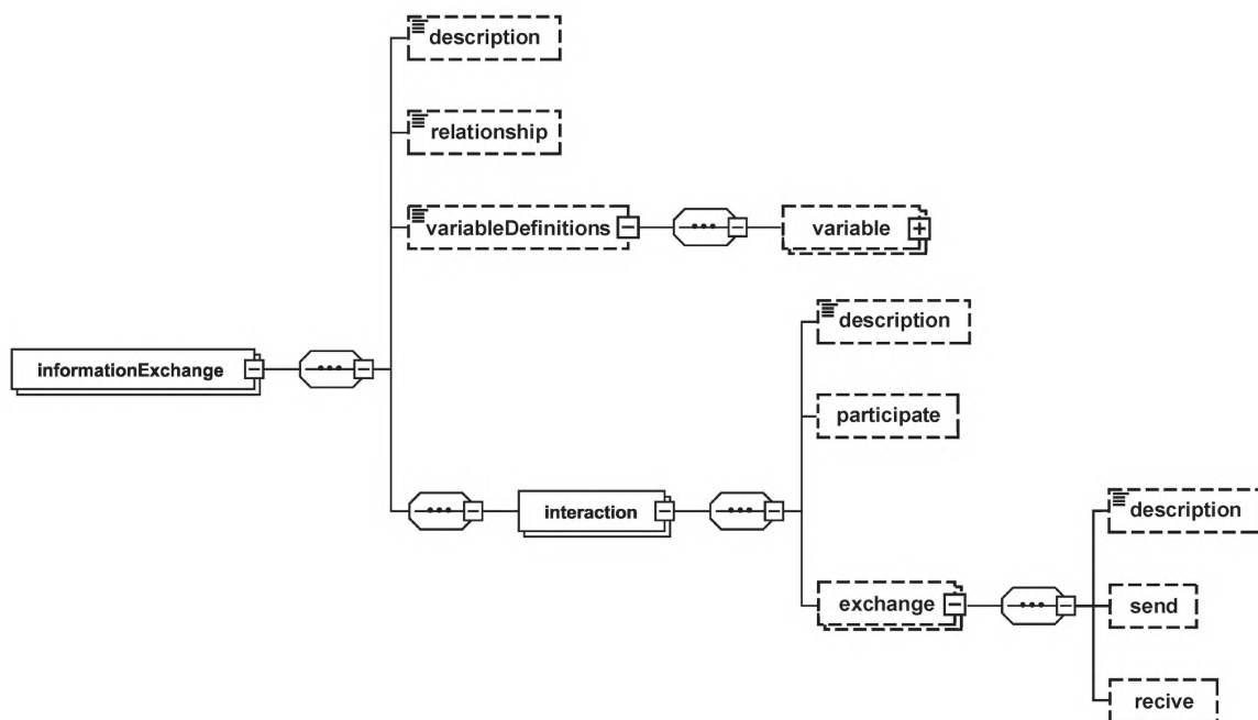
Рисунок 13 — Графическое представление элемента ADM-матрицы InformationExchange
