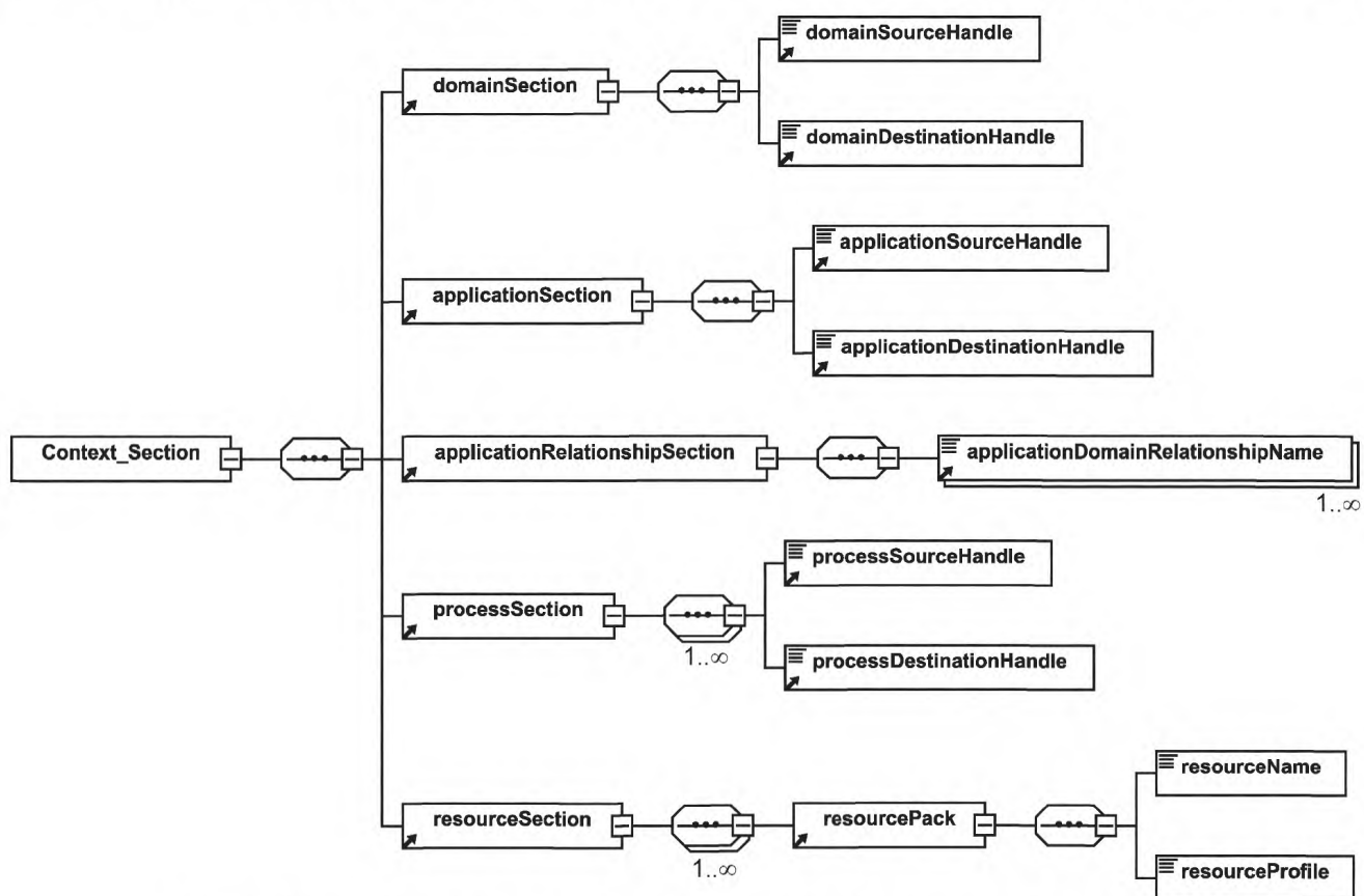
Рисунок 6 — Графическое представление элемента AIM-матрицы Context_Section
