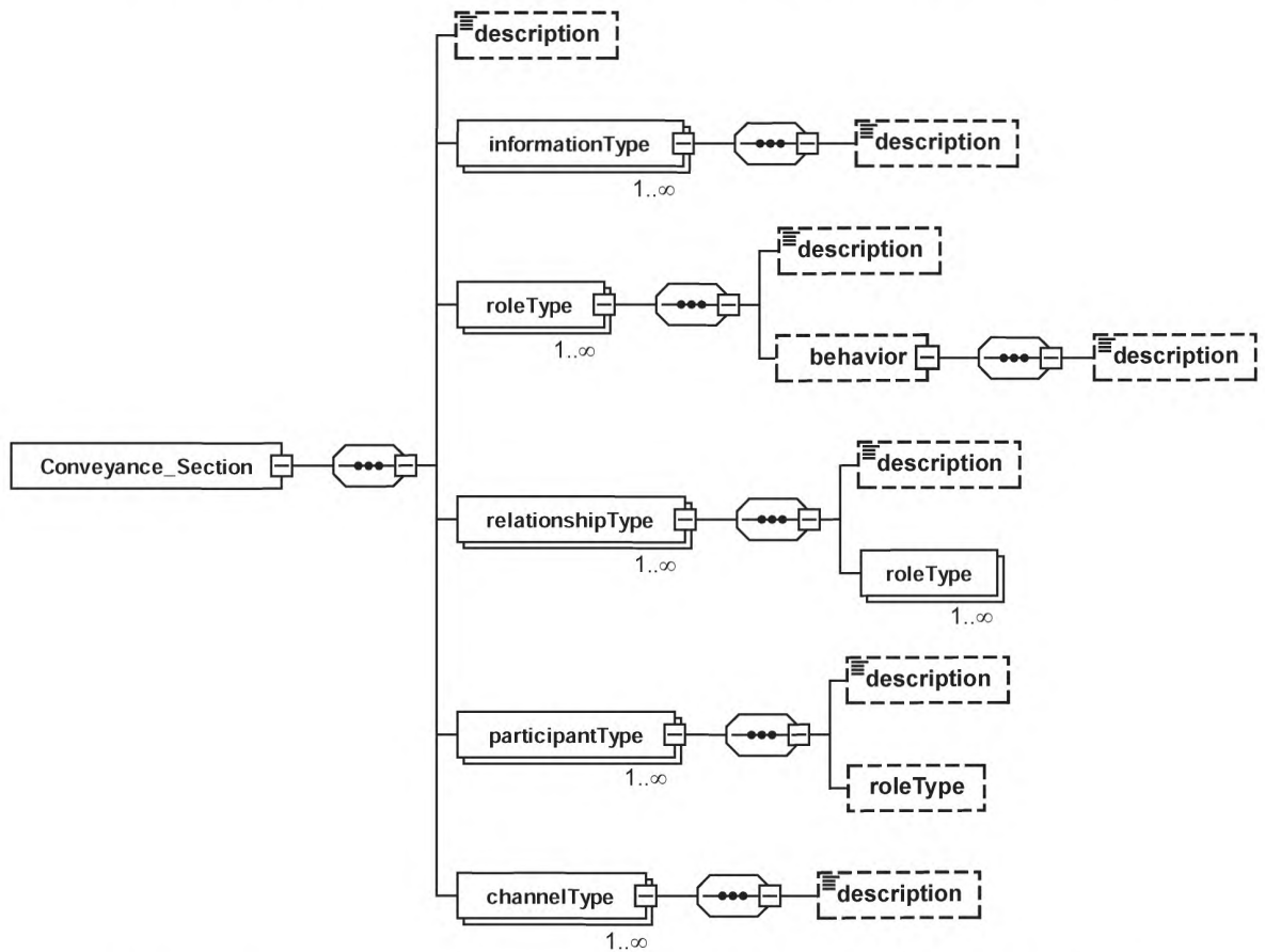
Рисунок 11 — Графическое представление элемента ADM-матрицы Conveyance_Section
