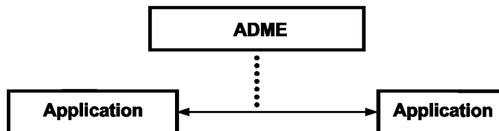
Рисунок 2 — Элементы ADM-матрицы
