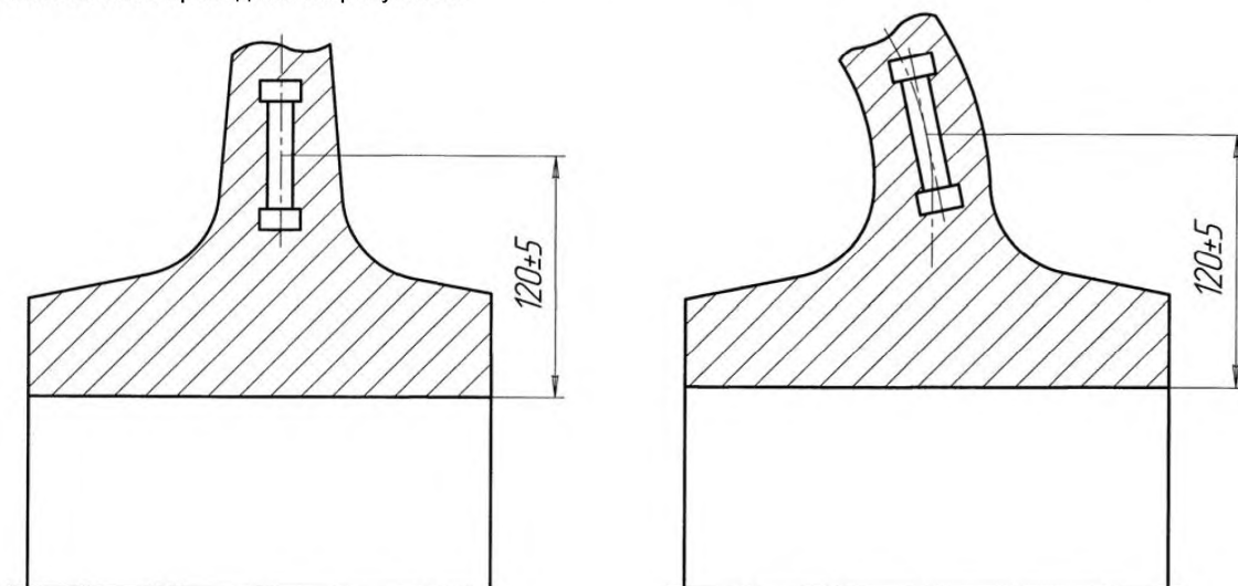
а) Центр с прямолинейным диском
