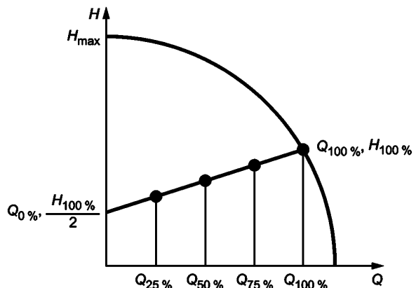
Рисунок 1 — Опорный график производительности циркуляционного насоса
