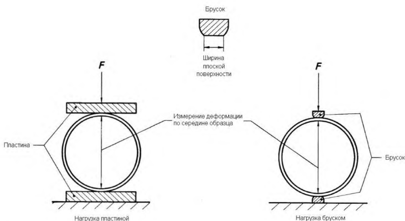
Рисунок 2 – Схема установки испытуемого образца в опорных площадках
