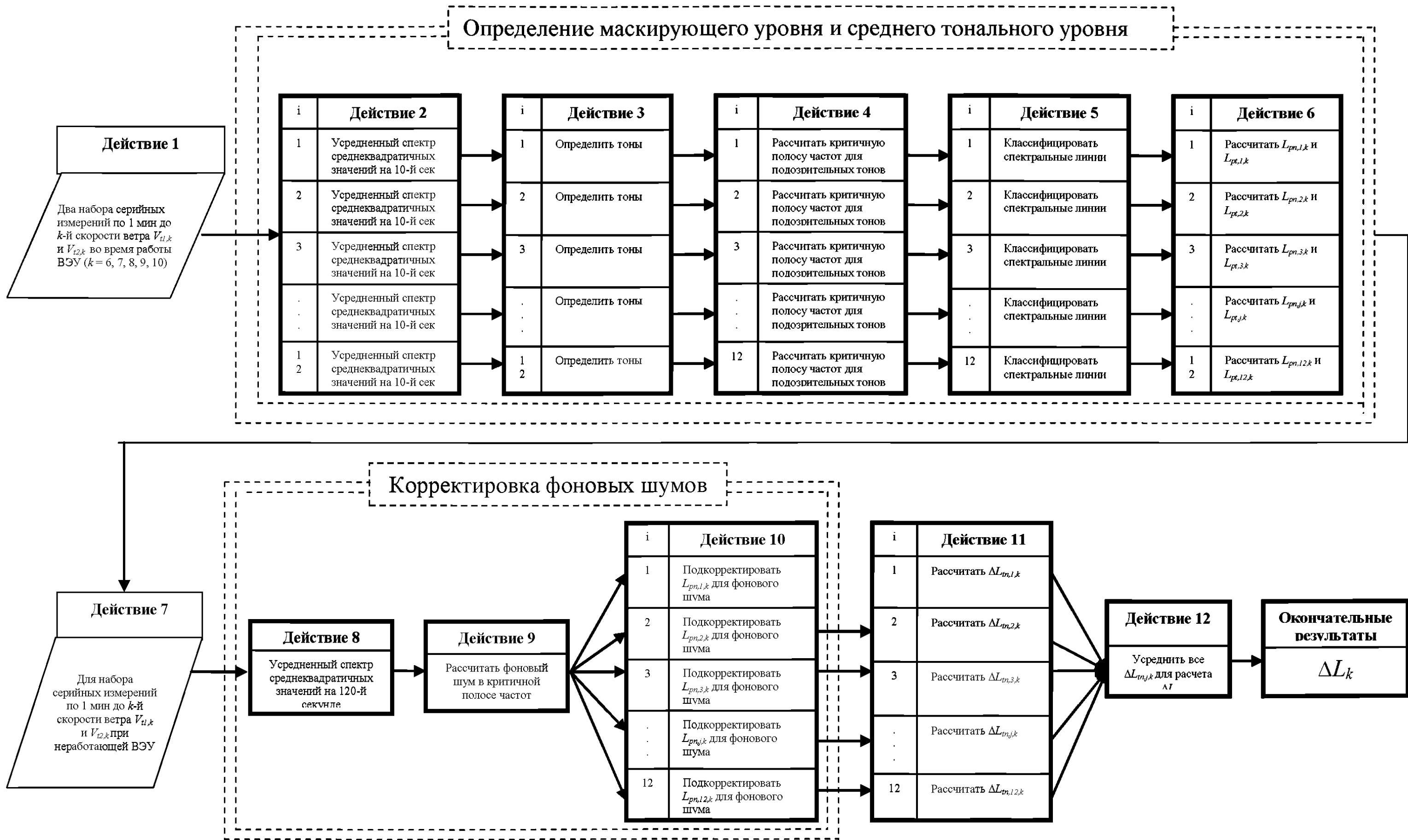
Рисунок 7 – Диаграмма последовательности операций для определения тональности
