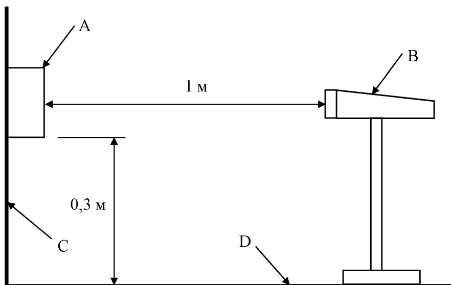
A — сигнализатор; B — микрофон; C — стена (вертикальная поверхность); D — пол или потолок (горизонтальная поверхность)
