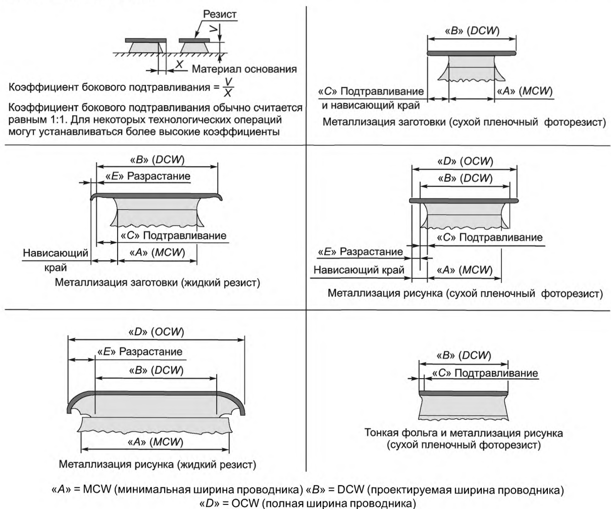
Рисунок 16 — Характеристика проводника
