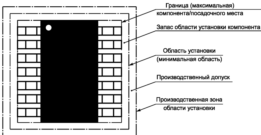
Рисунок 5 — Положение границы области установки
