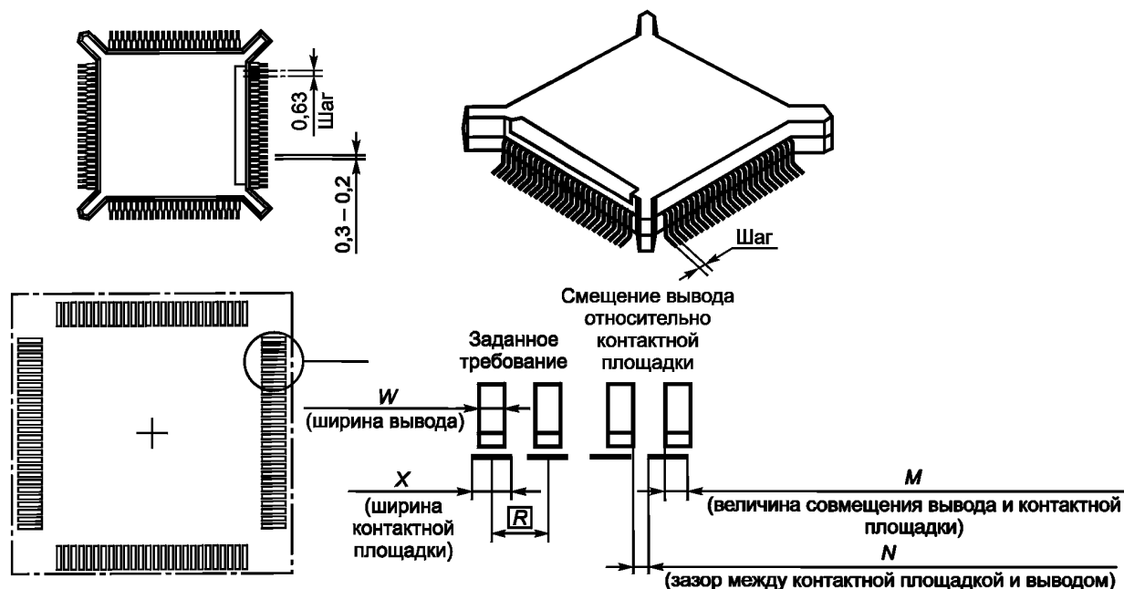
Рисунок 4 — Шаг для многывыводных компонентов
