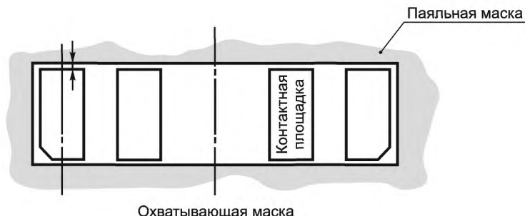
Рисунок 22 — Групповое освобождение от паяльной маски
