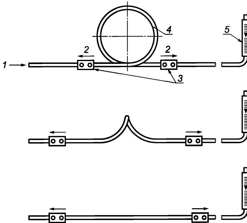
1 – подача воздуха, 2 – направление движения, 3 – зажимы, 4 – шланг, 5 – ротаметр
