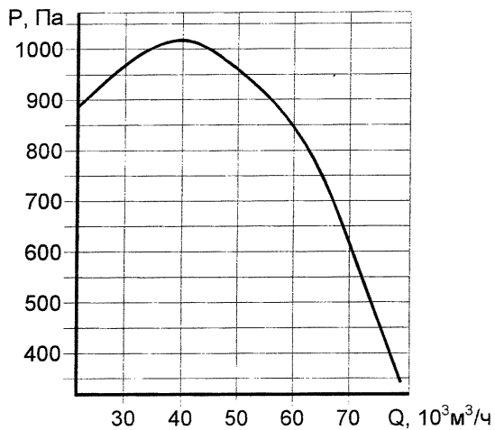
Рисунок 13 – Аэродинамическая характеристика вентилятора ВКРВ 10ДУ-10
