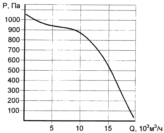
Рисунок 23 – Аэродинамическая характеристика вентилятора ВКРН 6,3ДУ-4
