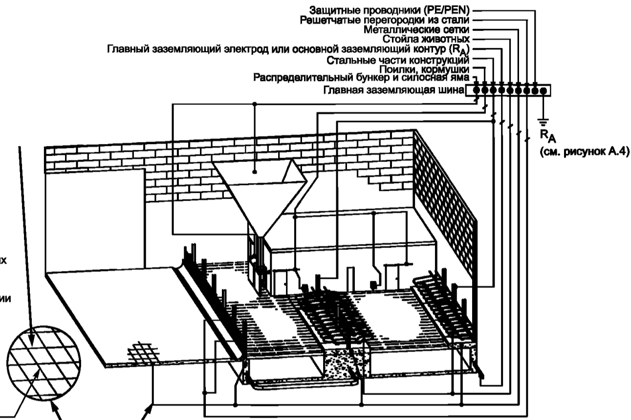
Рисунок А1 — Пример уравнивания потенциалов в коровнике
