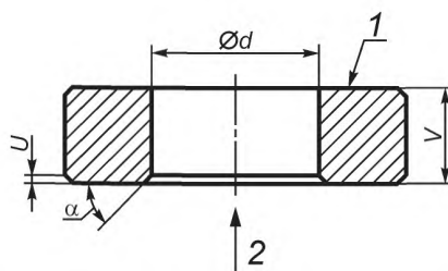
1 — поверхность X; 2 — направление введения цоколя
