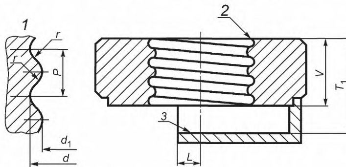
1 — деталь резьбы (правая резьба); 2 — острая часть кромки резьбы; 3 — поверхность X
