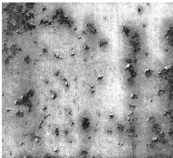
Рисунок 12 — Коррозия металла балл К4 (или R/4)
