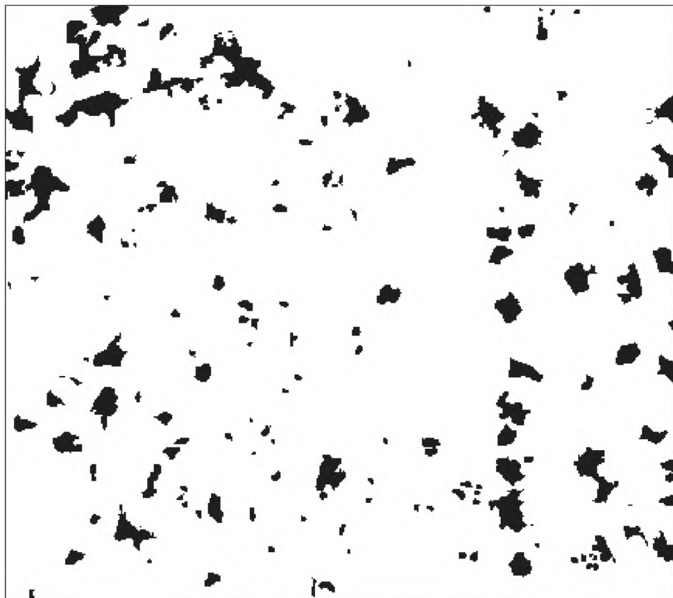
Рисунок Ж.4 — Коррозия металла, балл К4 (или R4)
