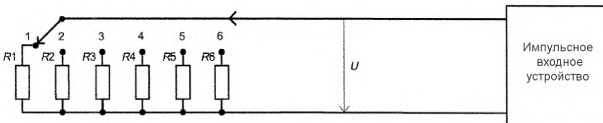
Рисунок Е.3 – Испытательная схема импульсного входного устройства
