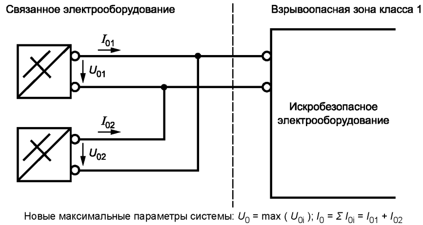
Рисунок В.2 – Параллельное соединение. Суммирование токов
